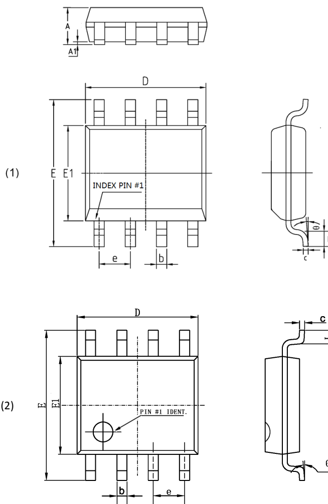
SOP 8 (150mil)
